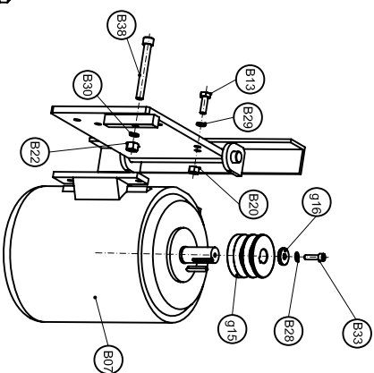
MOTOR SUB_ASSY
